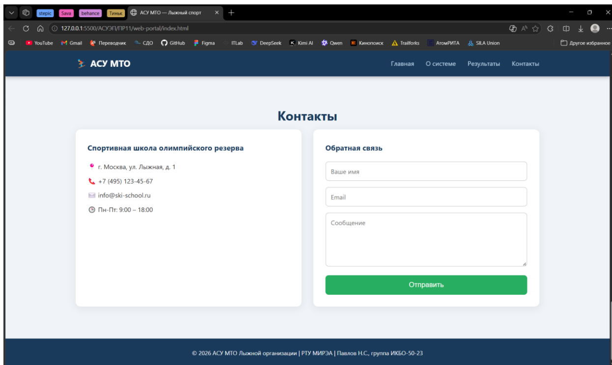
Рисунок 5.8 – Раздел «Контакты»
