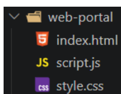
Рисунок 2.1 – Файловая структура
